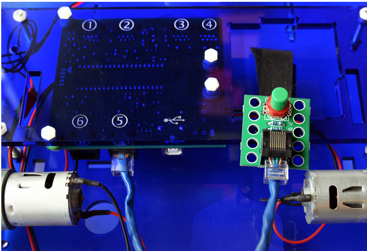
Figura 2.1.C: Sensor conectado al robot
