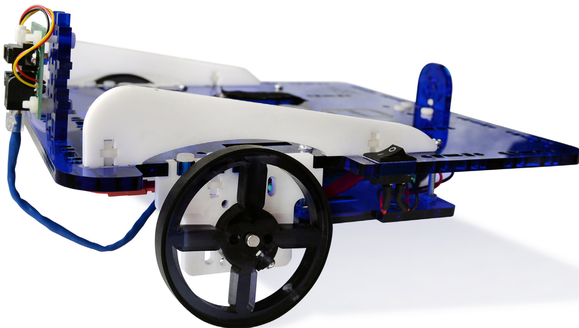
Figura 3.3.2.A: Robot con sensor distancia apuntando hacia adelante
