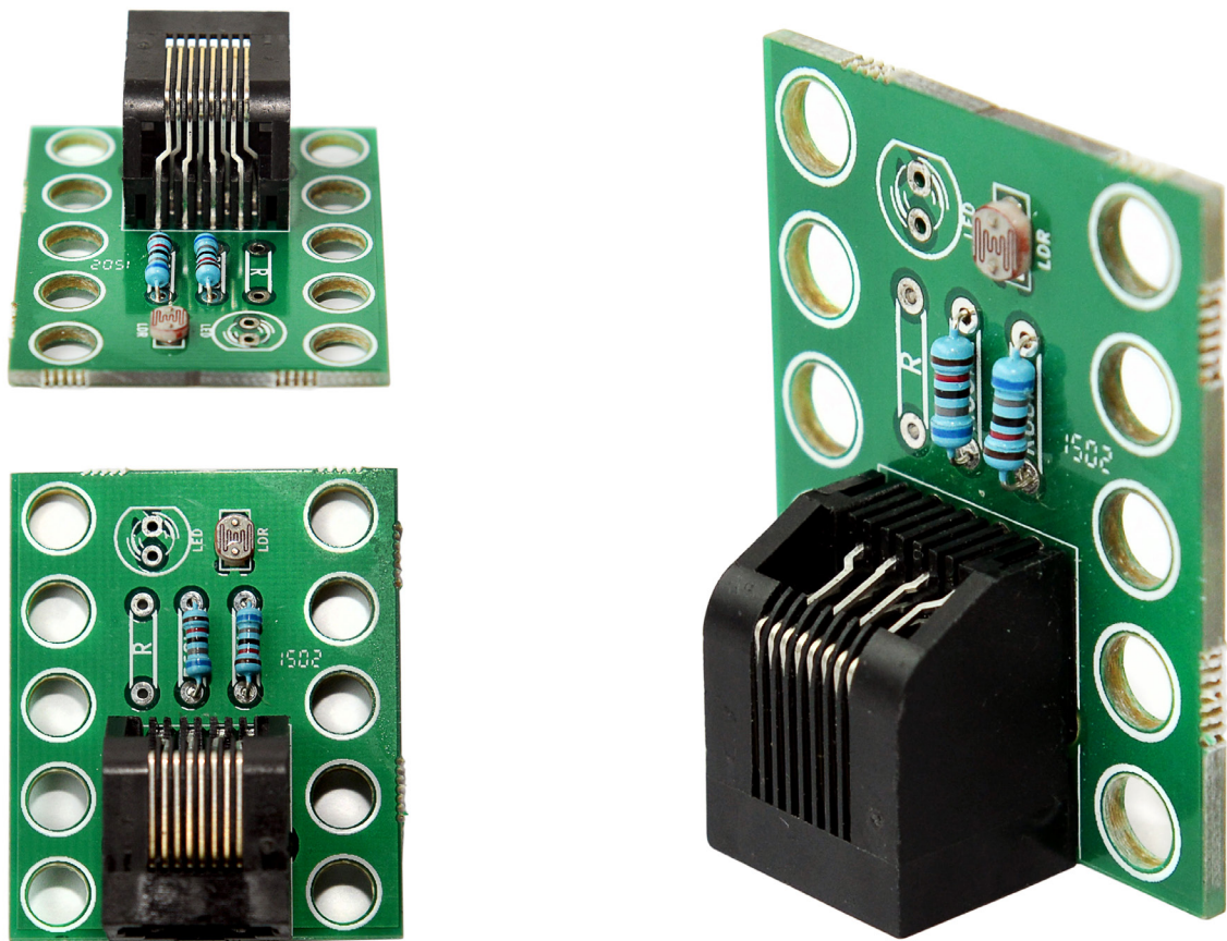
Figura 2.5.A: Sensor de luz
