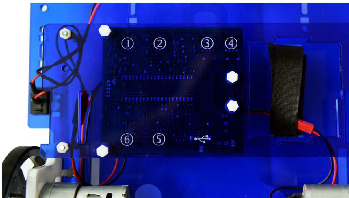
Figura 2.1.A: Chasis y puertos del robot Butiá
